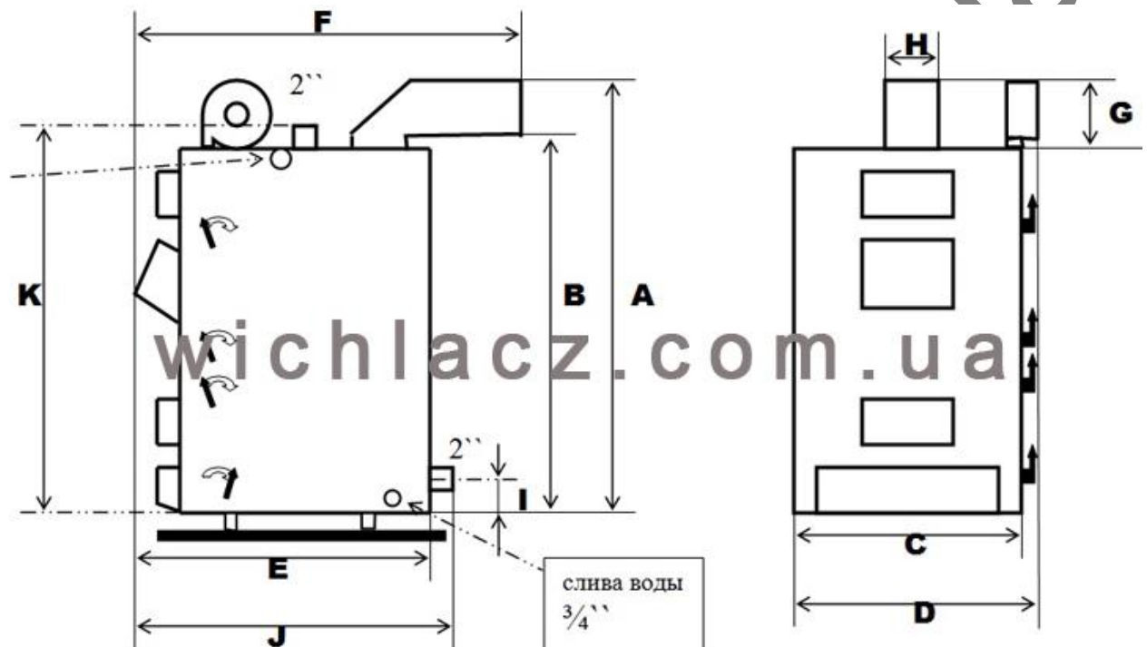
Рисунок 1 – Габаритне креслення котла типу GK-1
